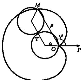
Рис. 2.22 Кардиоида. Из равенства \sim TM = \sim TO выведите уравнение p = 2a(1 - \cos \varphi)
