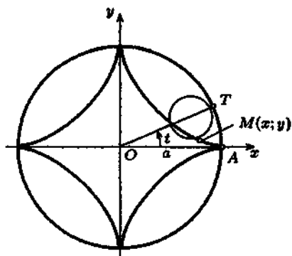
Рис. 2.21 Астроида. Из равенства \sim TM = \sim TA выведите уравнения x = a \cos^3 t , y = a \sin^3 t
