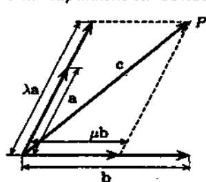
Рис. 7.11 \mathbf{c} = \lambda \mathbf{a} + \mu \mathbf{b} .
